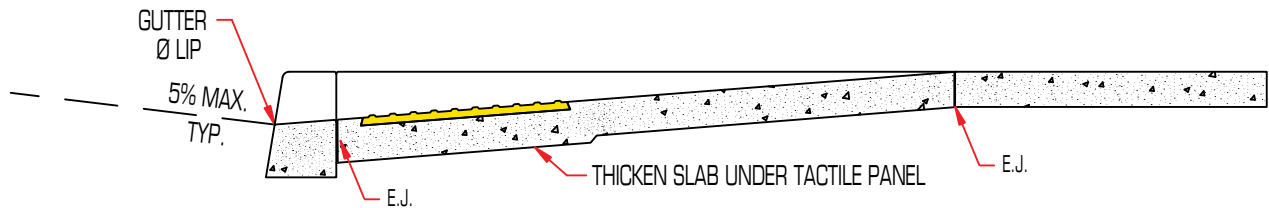
SECTION A-A
